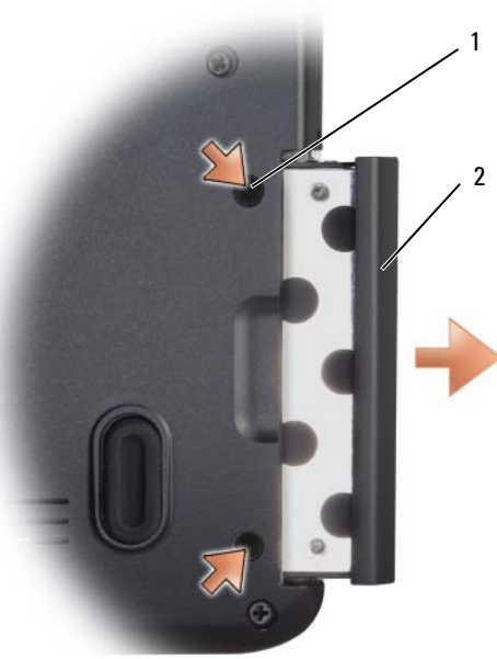
1 螺钉 (2) 2 硬盘驱动器
