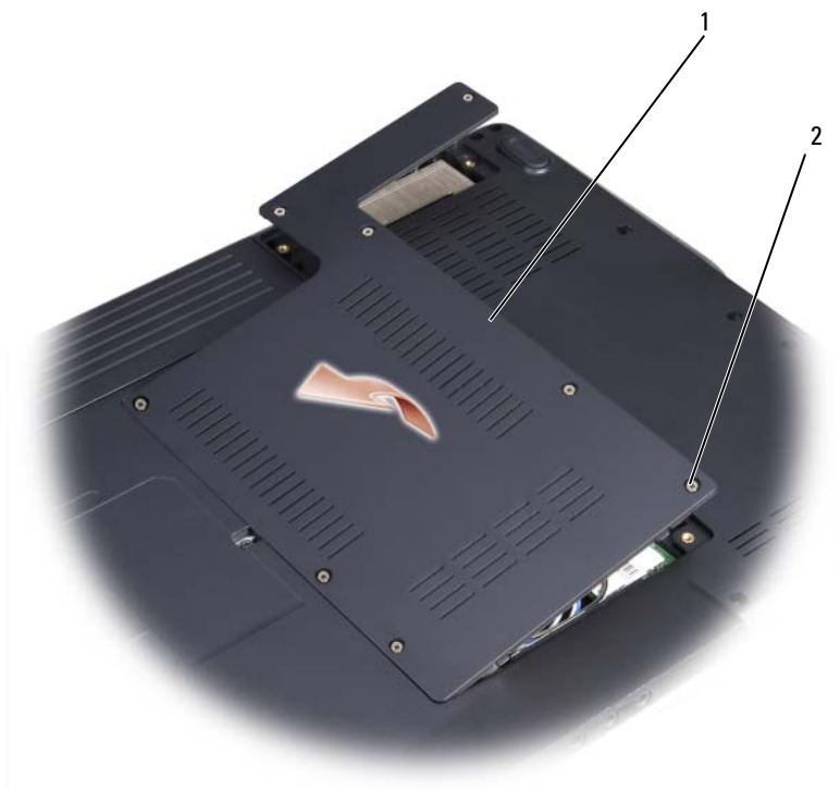
1 护盖 2 固定螺钉(5)
